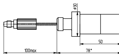
Рисунок 2 - ПЭП типа ПЭП-3-50
