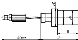
Рисунок 2 г - ПЭП типа ПЭП-3-35
