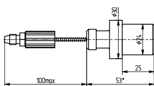
Рисунок 2 в - ПЭП типа ПЭП-3-25
