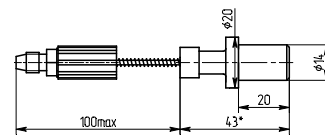
Рисунок 2 ж - ПЭП типа ПЭП-6-20
