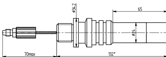
Рисунок 2 е - ПЭП типа ПЭП-3-65
